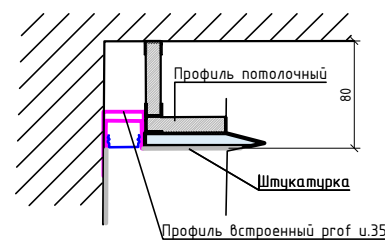
Разрез 3-3
