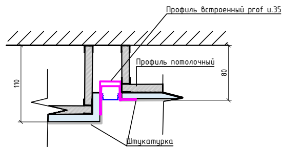
Разрез 2-2
